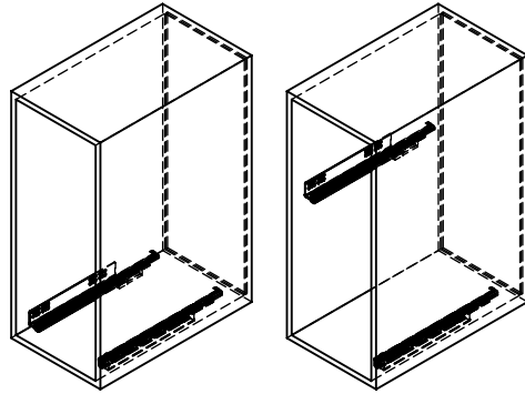
2. Варианты установки направляющих
